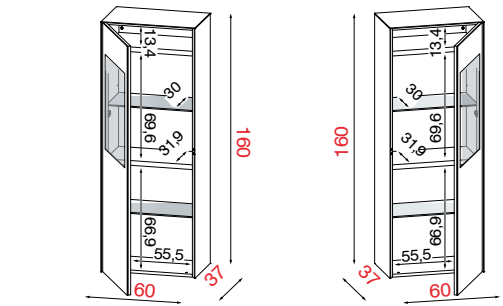
Li = Drehtür mit Linksanschlag
