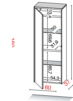
Li = Drehtür mit Linksanschlag
