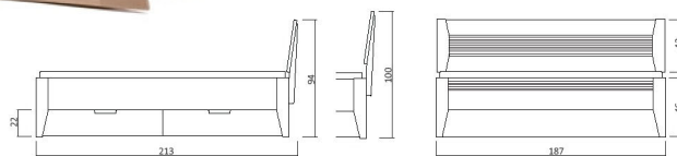
Bsp. Außenmaße (cm) Bettgröße 180x200
