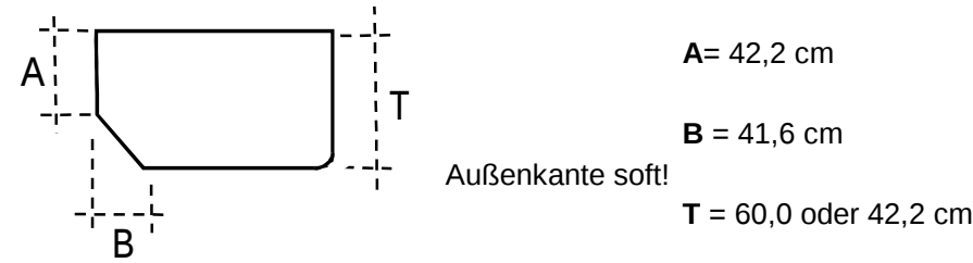
Detail Arbeitsplatte
