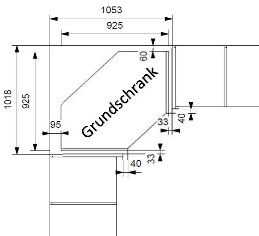
45° Ecke, 1-türig
