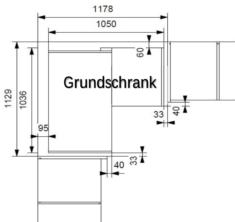
90° Ecke, 2-türig
