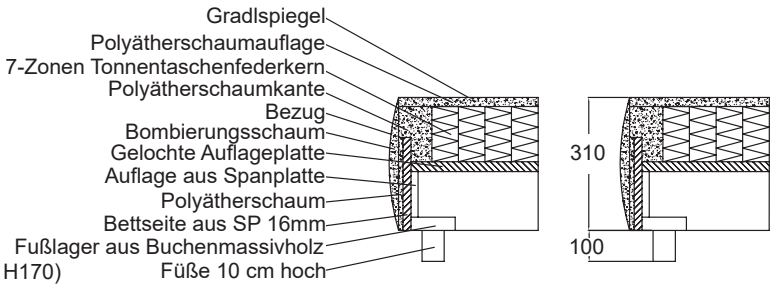
Querschnittansicht Boxunterbau SC56:
