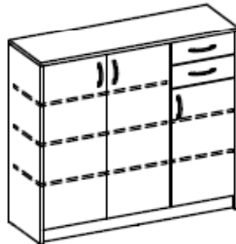
38-006-.. Kommode 6 hoch 3 Türen, 2 SK 2 kl. + 3 gr. E-Böden 109 x 112 x 35 cm
