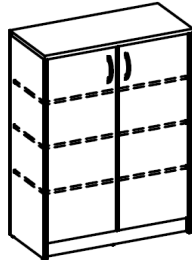
38-002-.. Kommode 2 hoch 2 Türen 3 E-Böden 74 x 112 x 35 cm
